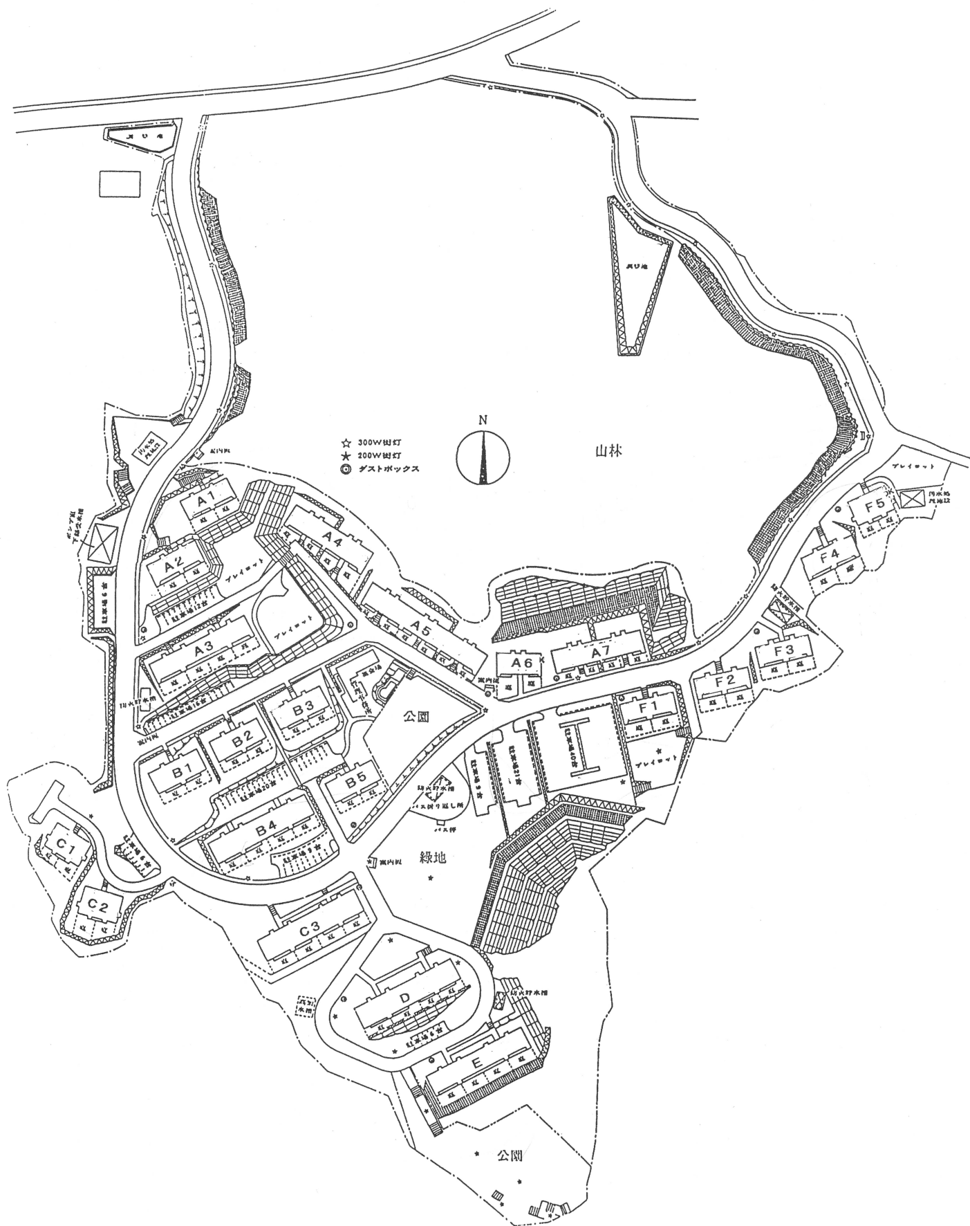
鎌倉グリーンハイツ配置図
